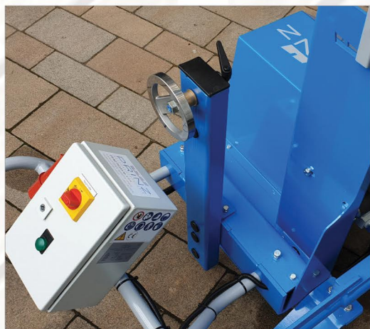
Mechanizm przesuwu lewo/prawo (opcja)
